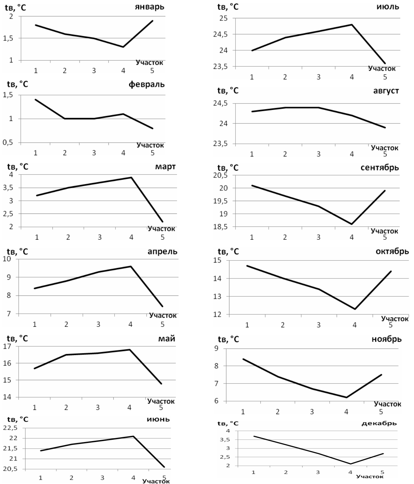
Рис. 8. Среднегоголетние температуры поверхности воды по месяцам на пяти участках Каховского водохранилища
