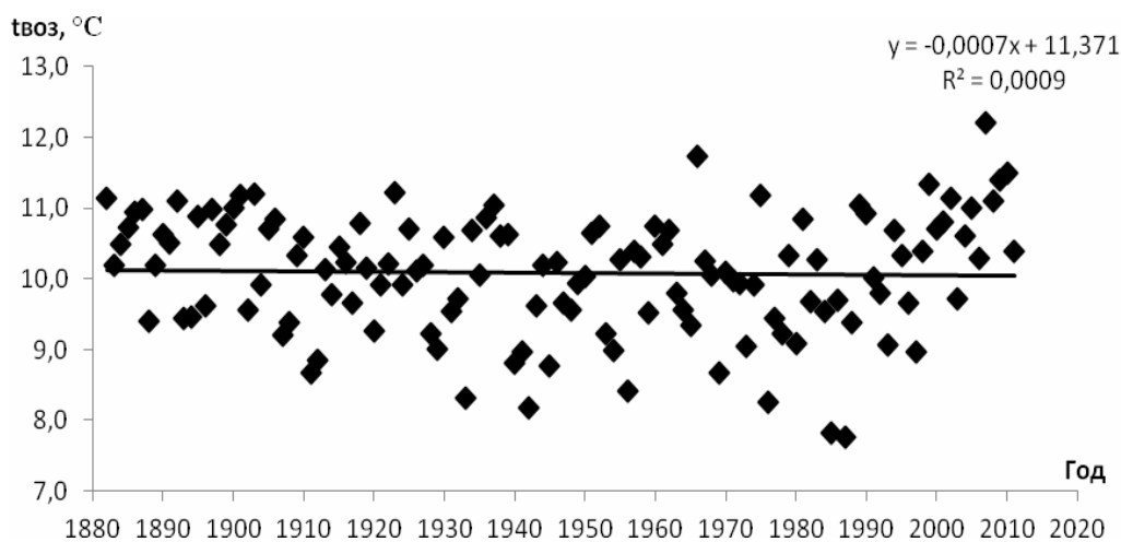
Рис. 3. Хронологический график температуры воздуха (г. Херсон)
