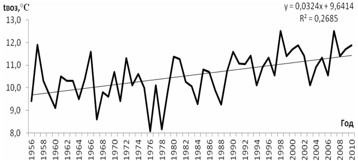
Рис. 2. Хронологический график среднегодовой температуры воздуха над акваторией Каховского водохранилища
