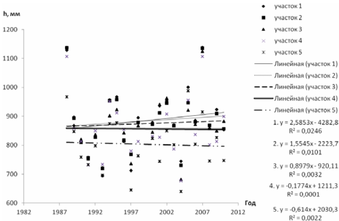
Рис. 7. Временная изменчивость среднегодового слоя испарения с водной поверхности участков акватории Каховского водохранилища
