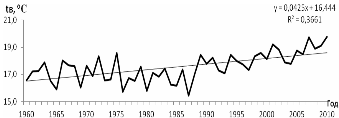
Рис. 4. Хронологический график среднегодовой температуры поверхности воды Каховского водохранилища
