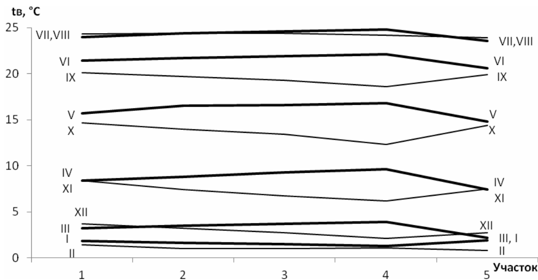
Рис. 9. Среднегодовья месячные температуры поверхности воды по месяцам на участках Каховского водохранилища за период 1988-2010 гг.
