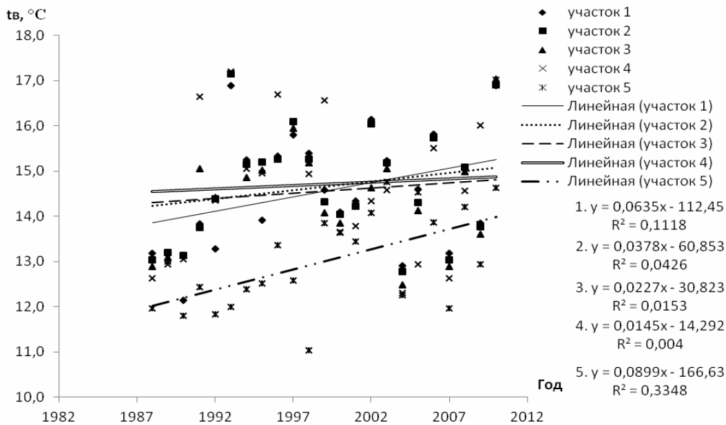
Рис. 6. Временная изменчивость среднегодовых температур воды на участках акватории Каховского водохранилища
