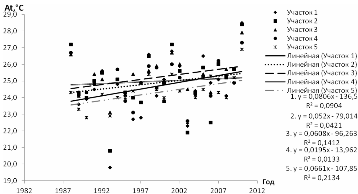
Рис. 13. Временная изменчивость среднегодовых амплитуд колебания температуры поверхности воды на участках Каховского водохранилища
