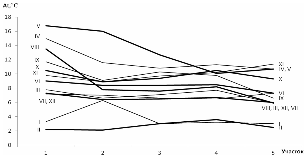
Рис. 11. Среднегодовое месячные амплитуды колебания температуры поверхности воды по участкам Каховского водохранилища за период 1988-2010 гг.
