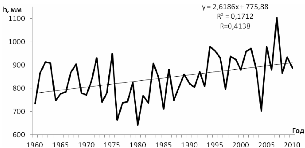
Рис. 5. Хронологический график среднегодового слоя испарения с поверхности воды Каховского водохранилища
