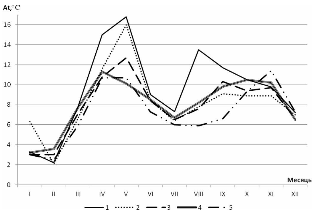
Рис. 10. Внутригодовое распределение среднееголетних амплитуд колебания температуры поверхности воды Каховского водохранилища за 1988-2010 гг.
