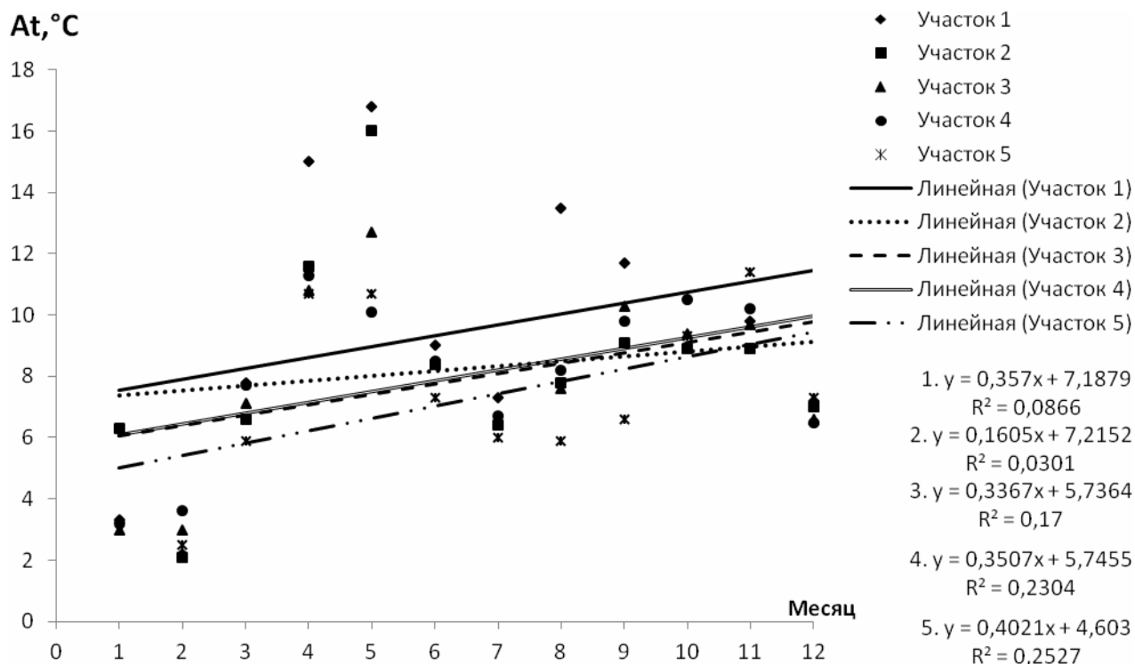
Рис. 12. Хронологический график изменений среднемесячных амплитуд колебания температуры поверхности воды на участках Каховского водохранилища
